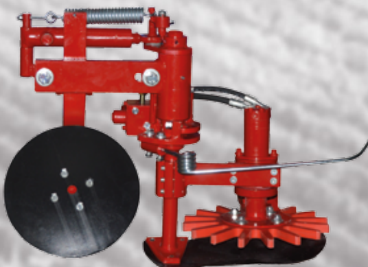
Stock-Kopier-Gerät mit Flachschar und Fingerhacke
