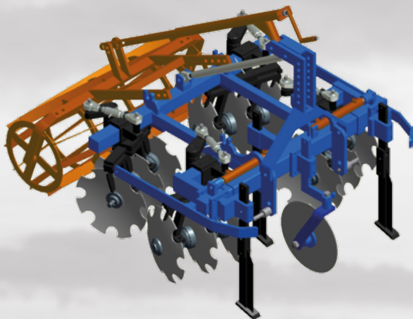
TKV Rahmen als Scheibenegge
