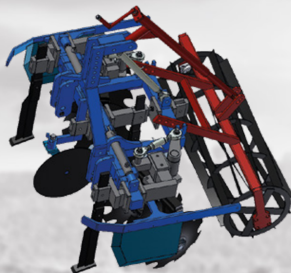
Geräterahmen und Kurzgrubber TKV Easy
