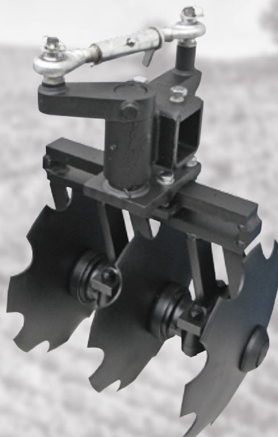
Scheibenwalzen 1 Paar mit 2 x 3 Scheiben gezackt
