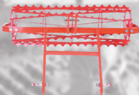
Krümelwalze Ø 400 mm mit Spindelverstellung
